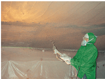
吹付け施工
